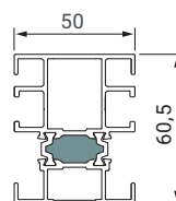
Verbreiterungsprofil VP 50
