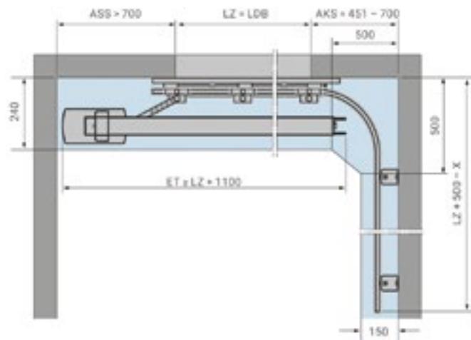
DS-Beschlag (Doppelschiene, Antrieb Deckenmontage B)
