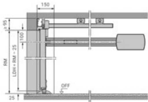
Antrieb Wandmontage
