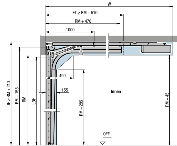
H-Beschlag
