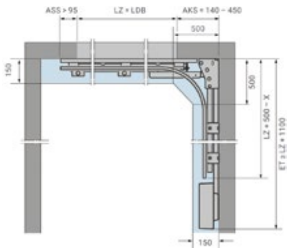
Bestimmung der Antriebsschiene (ES- und DS-Beschlag)
