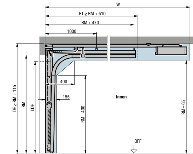
L-Beschlag
