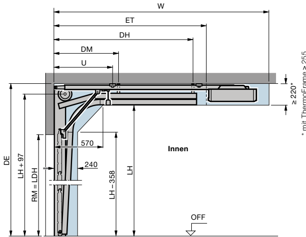
H-Beschlag
