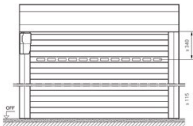
Einbau hinten / in der Öffnung - Innen-Rolltor
