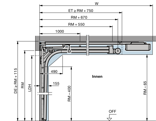
L-Beschlag
