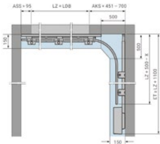
ES-Beschlag (Einfachschiene, Antrieb Wandmontage)
